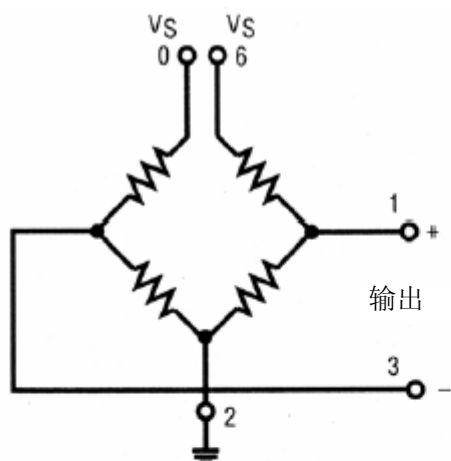
图 1 等效电路
